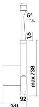
Vista lateral de la instalación con motor trasero
