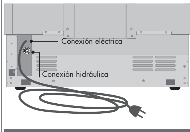
FIG.1 - PARTE DE ATRÁS DEL EQUIPO
