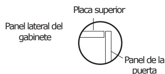
Referencia e indicación del tamaño de la puerta superpuesta completa
