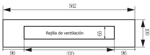
Diagrama esquemático del zócalo
