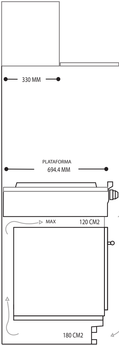
VISTA LATERAL
